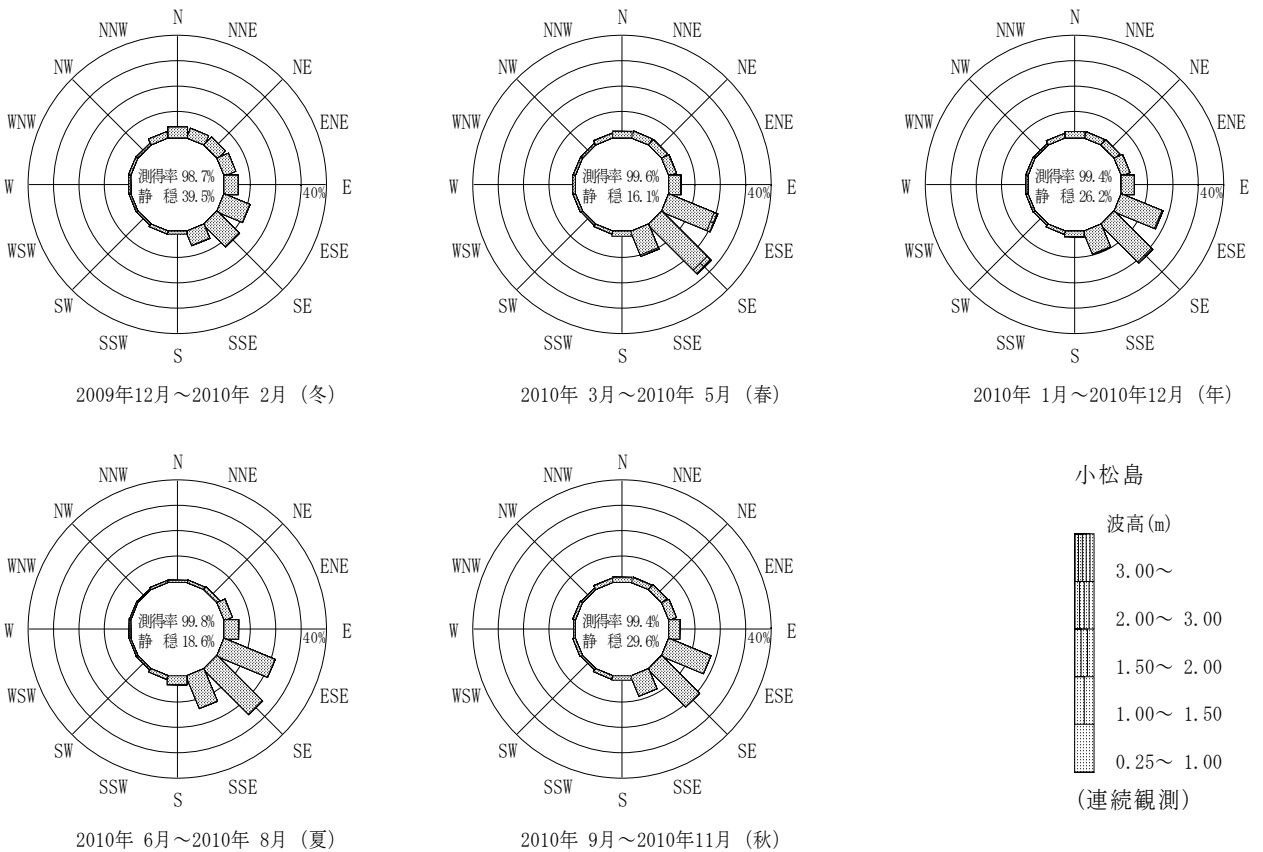
付図-B.2.51 小松島 波高・波向別出現頻度図(連続観測)
