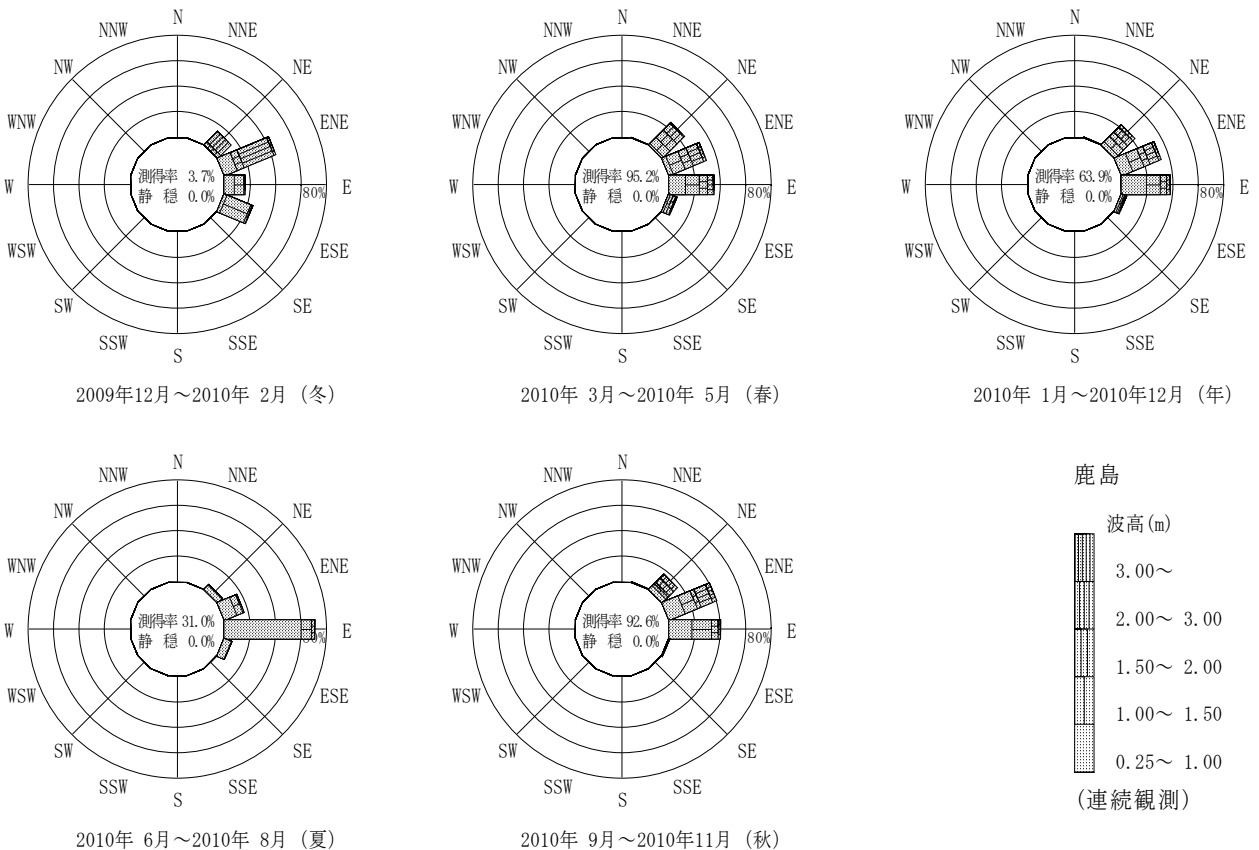
付図-B.2.41 鹿島 波高・波向別出現頻度図（連続観測）
