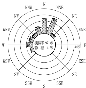
付図-A.2.20 浜田 波高・波向別出現頻度図
