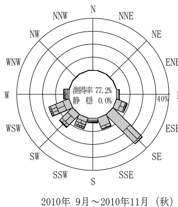
付図-A.2.49 潮岬 波高・波向別出現頻度図
