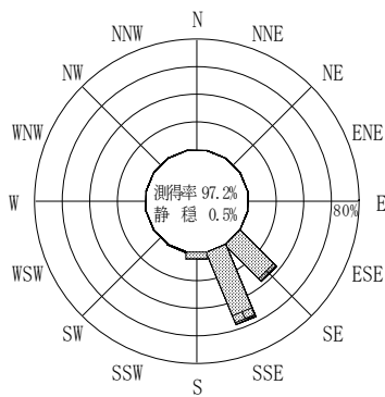
付図-A.2.36 石巻 波高・波向別出現頻度図
