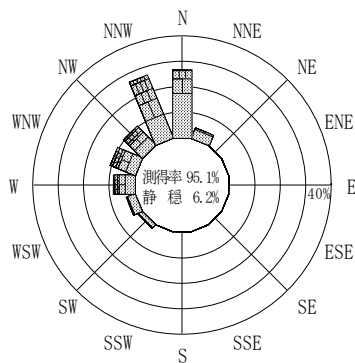
付図-A.2.14 福井 波高・波向別出現頻度図
