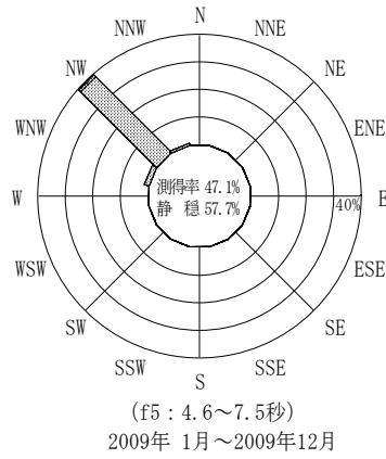
付図-A.3.61 石垣沖 波高・波向別出現頻度図 (f2, f3, f4, f5, 全周期帯)
