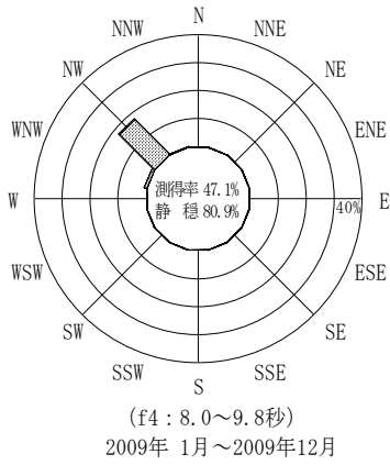
付図-A.3.61 石垣沖 波高・波向別出現頻度図 (f2, f3, f4, f5, 全周期帯)
