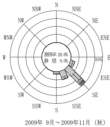
付図-B.2.47 御前崎 波高・波向別出現頻度図（連続観測）
