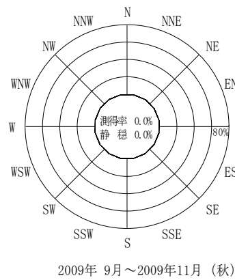
付図-B.2.31 むつ小川原 波高・波向別出現頻度図（連続観測）
