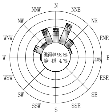
付図-A.2.18 鳥取 波高・波向別出現頻度図
