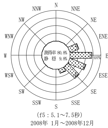
付図-B.3.59 中城湾 波高・波向別出現頻度図(連続観測, f2, f3, f4, f5, 全周期帯)
