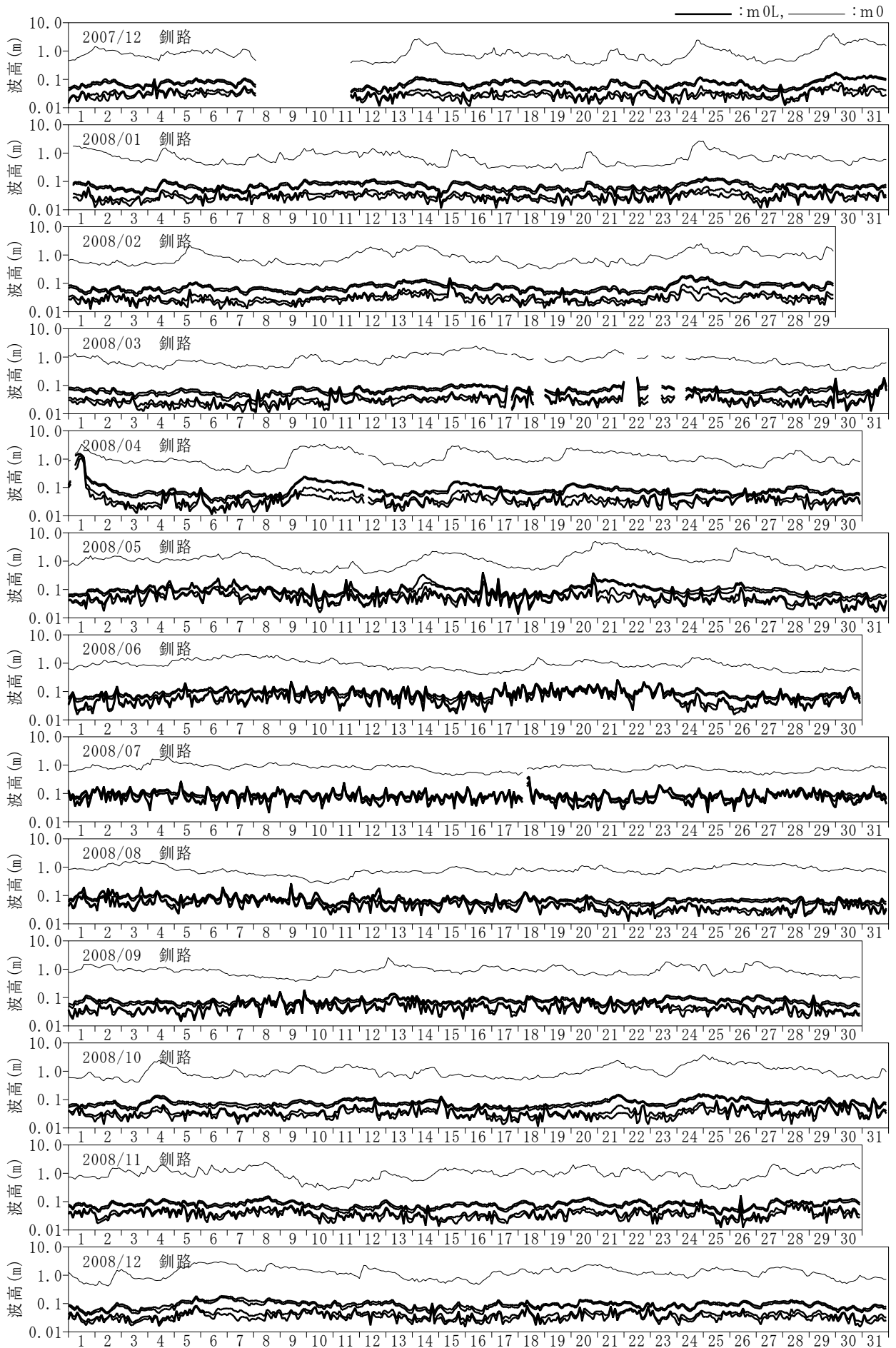
付図-C.1.28 長周期波高の経時変化図（釧路）
