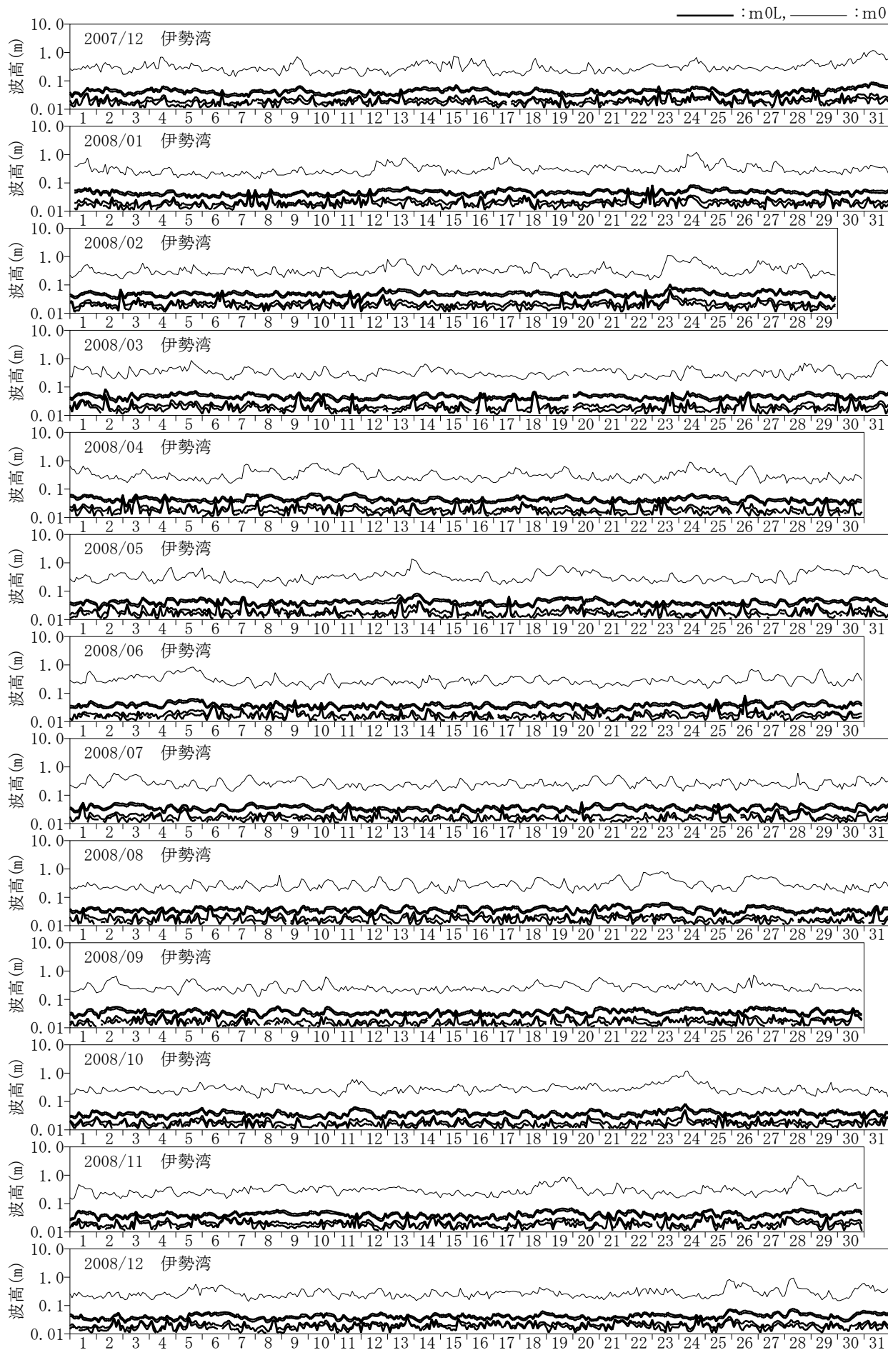
付図-C.1.48 長周期波高の経時変化図 (伊勢湾)
