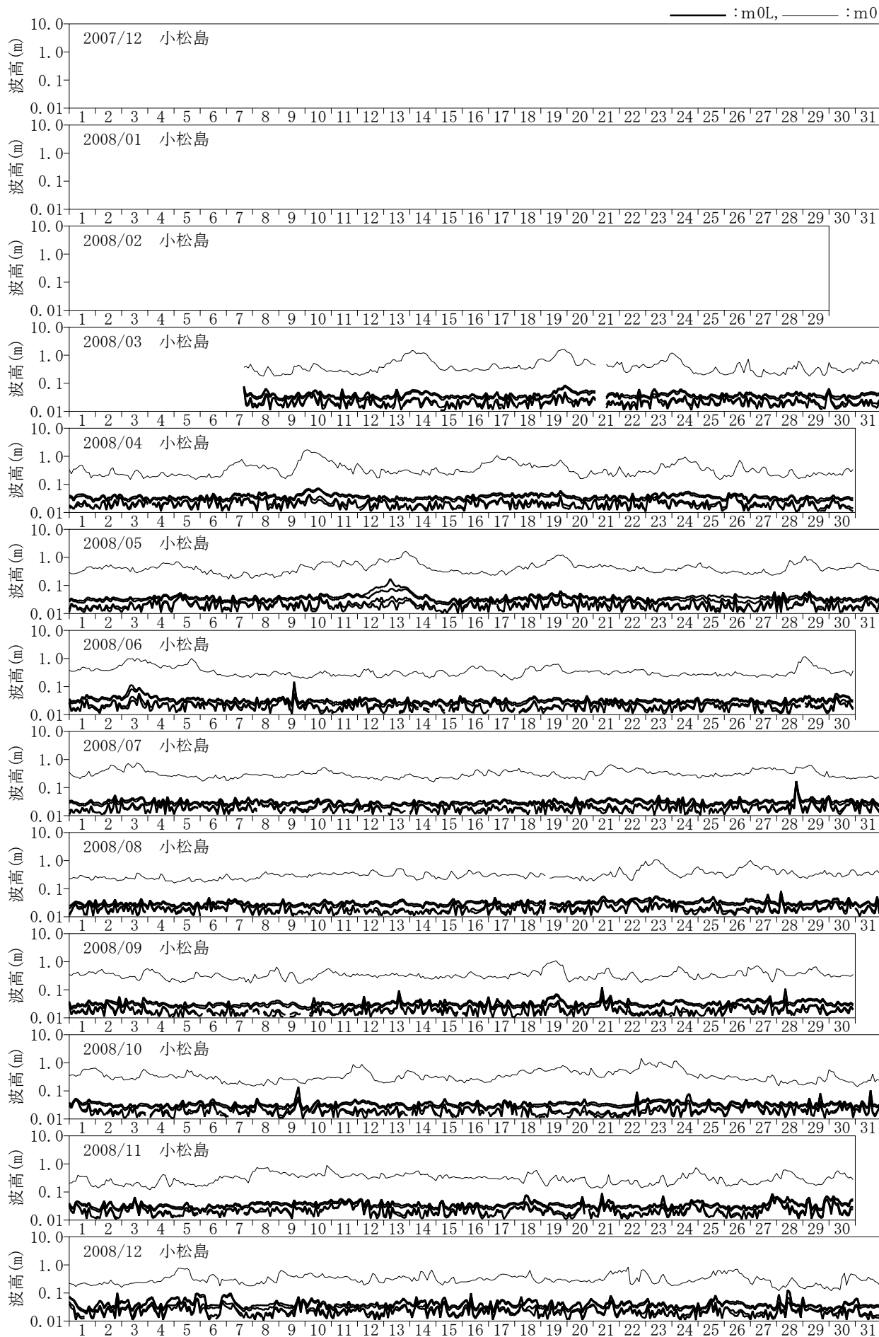
付図-C.1.51 長周期波高の経時変化図 (小松島)
