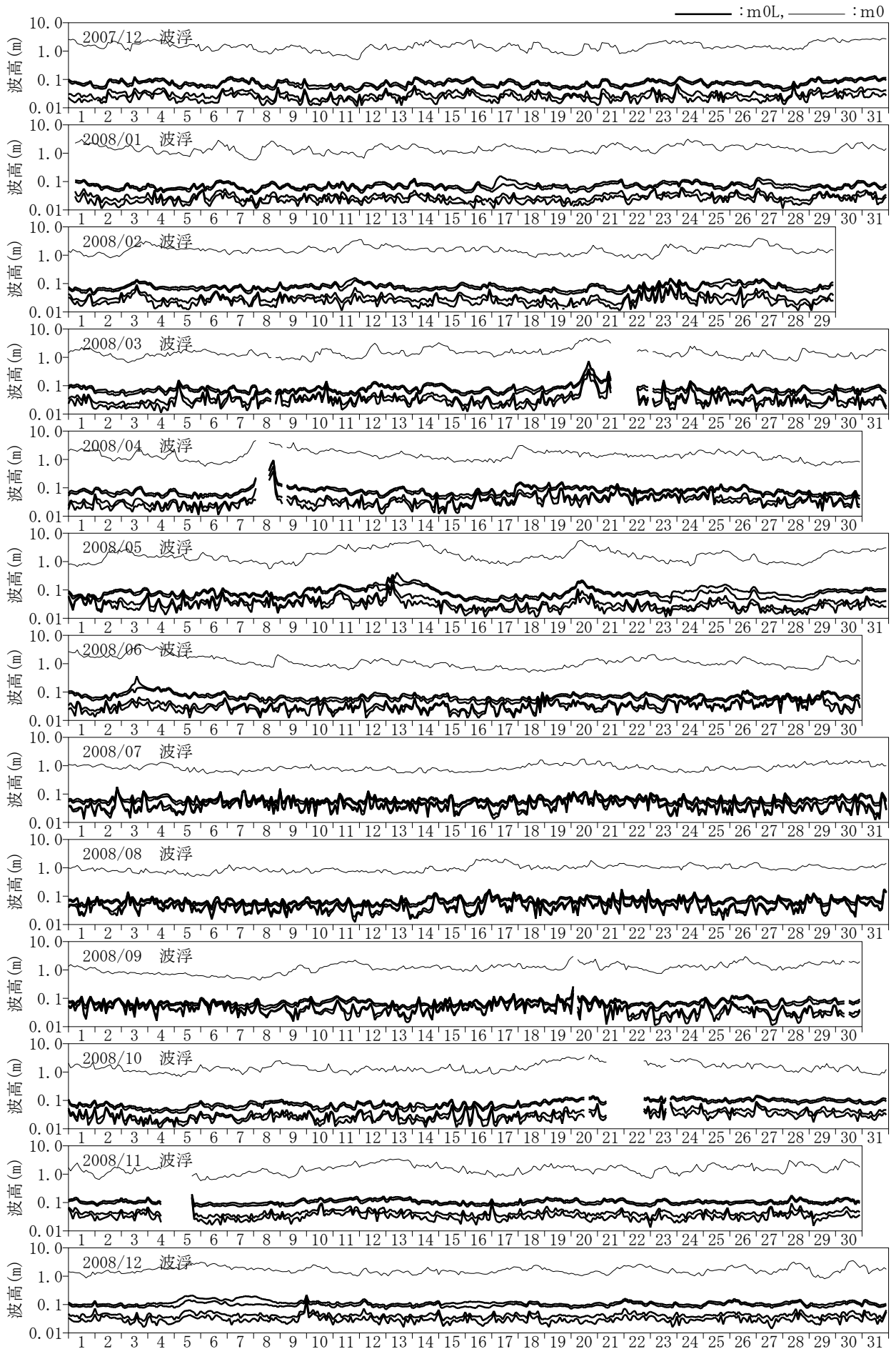
付図-C.1.44 長周期波高の経時変化図 (波浮)
