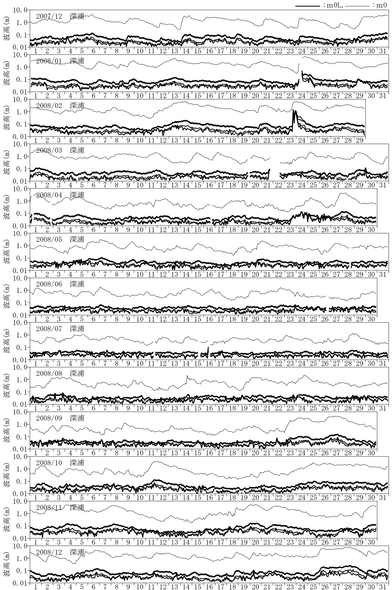
付図-C.1.5 長周期波高の経時変化図 (深浦)
