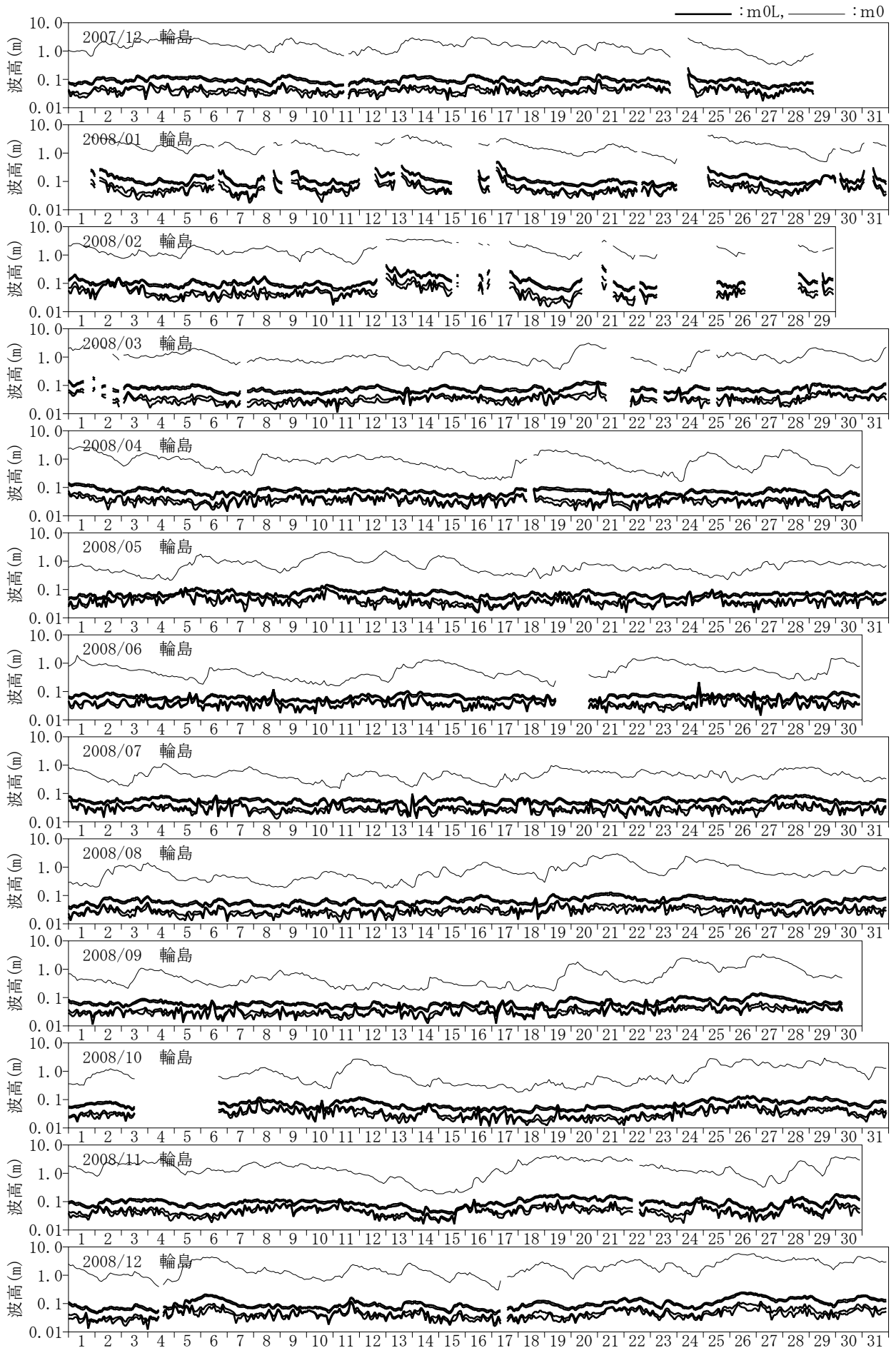
付図-C.1.12 長周期波高の経時変化図 (輪島)
