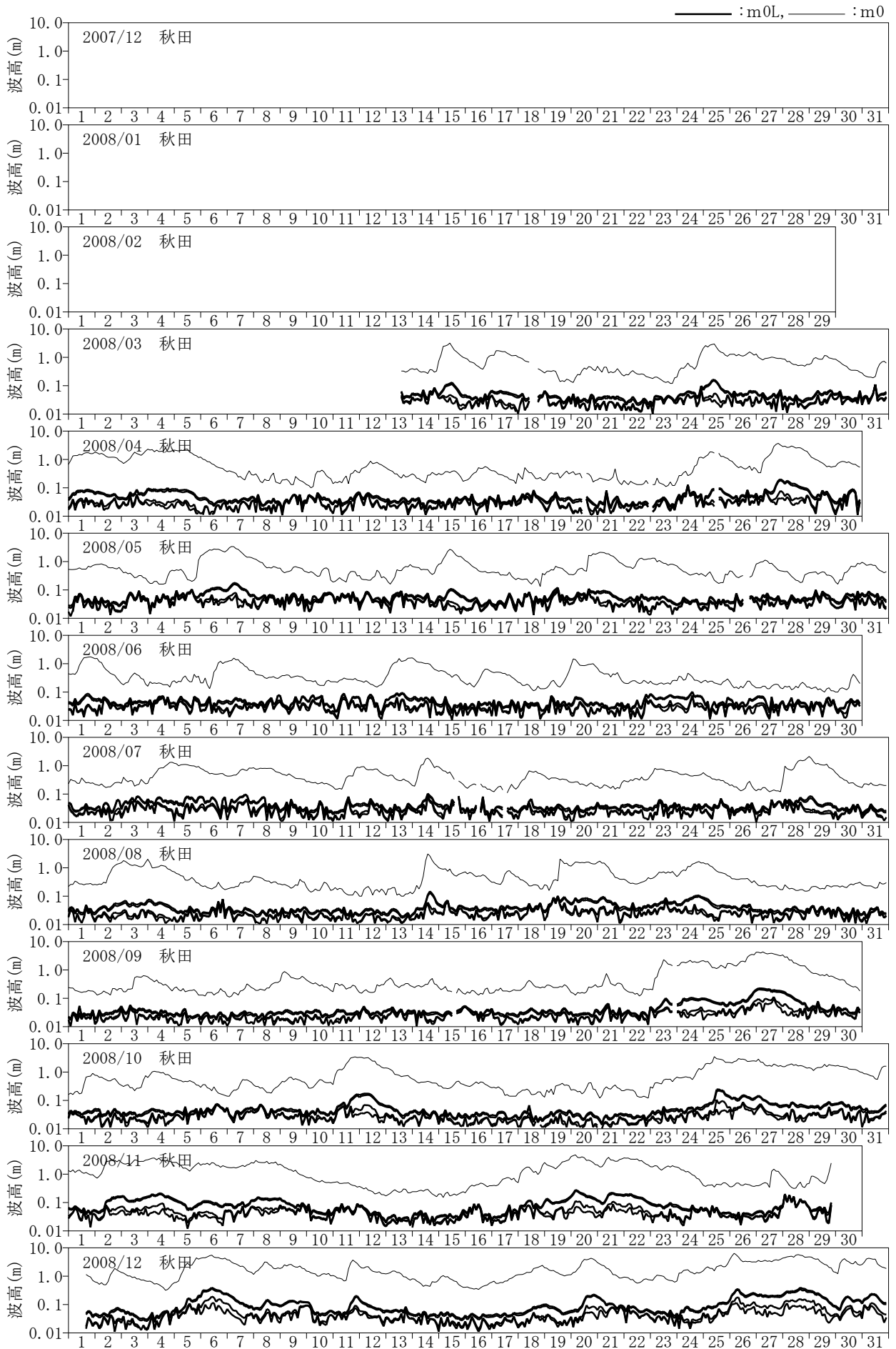
付図-C.1.6 長周期波高の経時変化図 (秋田)
