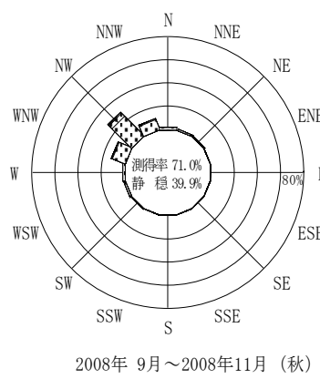
付図-B.2.61 石垣沖 波高・波向別出現頻度図（連続観測）
