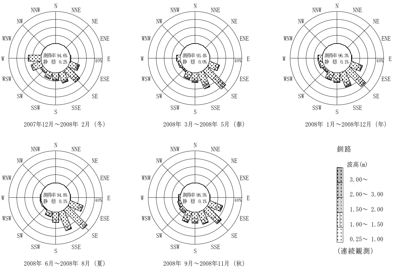
付図-B.2.28 釧路 波高・波向別出現頻度図（連続観測）
