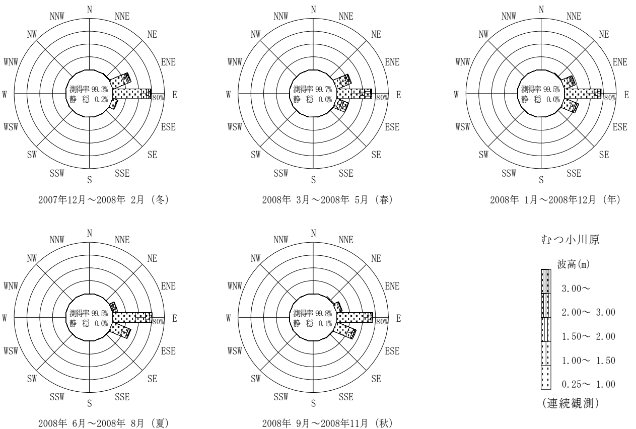
付図-B.2.31 むつ小川原 波高・波向別出現頻度図（連続観測）
