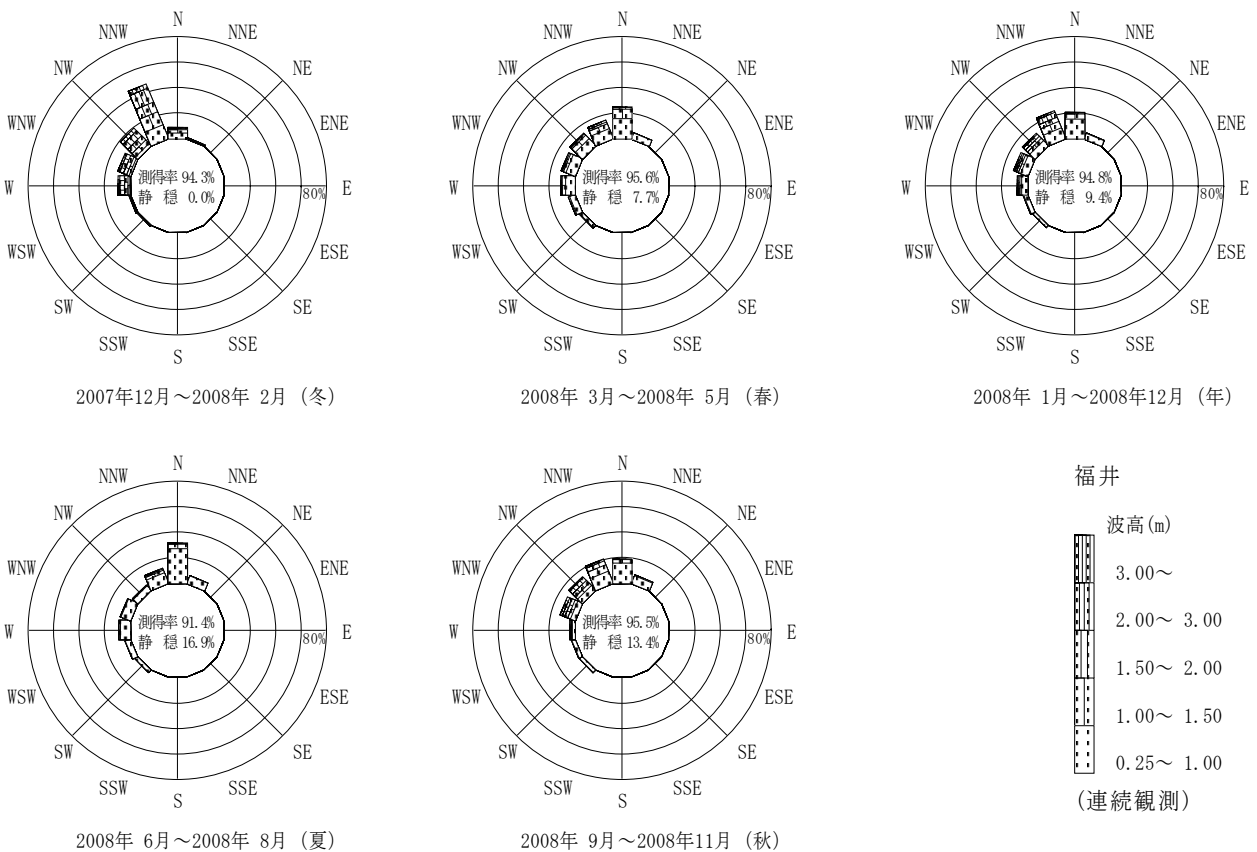
付図-B.2.14 福井 波高・波向別出現頻度図（連続観測）
