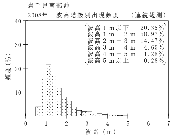
付図-B.1.62 岩手県南部沖 波候特性図 (連続観測)
