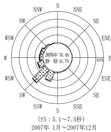
付図-B. 4. 23 伊王島 波高・波向別出現頻度図(連続観測, f2, f3, f4, f5, 全周期帯)
