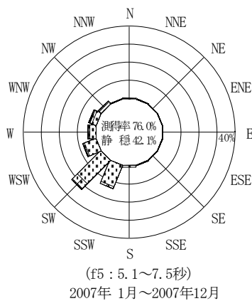
付図-A.4.23 伊王島 波高・波向別出現頻度図 (f2, f3, f4, f5, 全周期帯)
