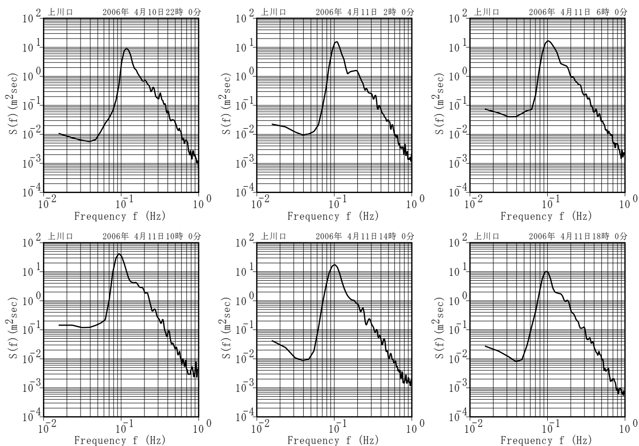
付図－A. 5. 54 上川口 代表的な高波期間中のスペクトル
