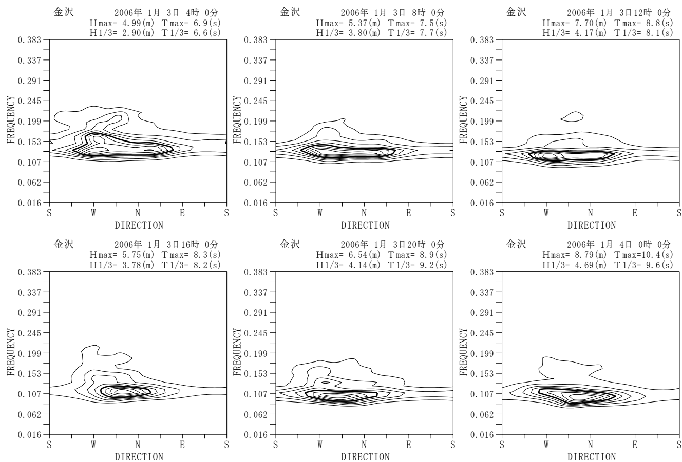
付図－A. 5. 13 金沢 代表的な高波期間中の方向スペクトル
