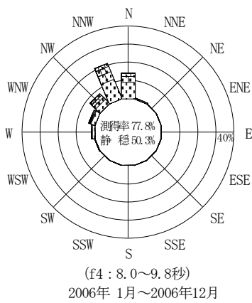
付図-A. 4. 13 金沢 波高・波向別出現頻度図 (f2, f3, f4, f5, 全周期帯)
