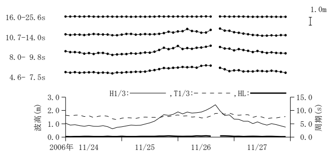
付図-A.3.54 上川口 周期帯別波浪特性の経時変化(高波期間中)
