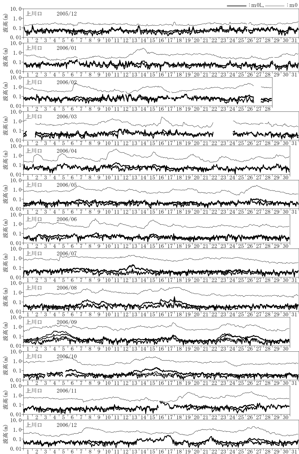
付図-C.1.54 長周期波高の経時変化図（上川口）
