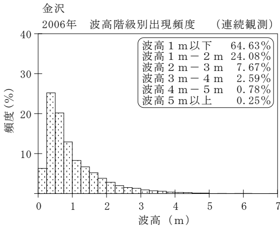
付図-B.1.13 金沢 波候特性図（連続観測）
