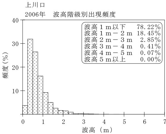
付図-A. 1. 54 上川口 波候特性図
