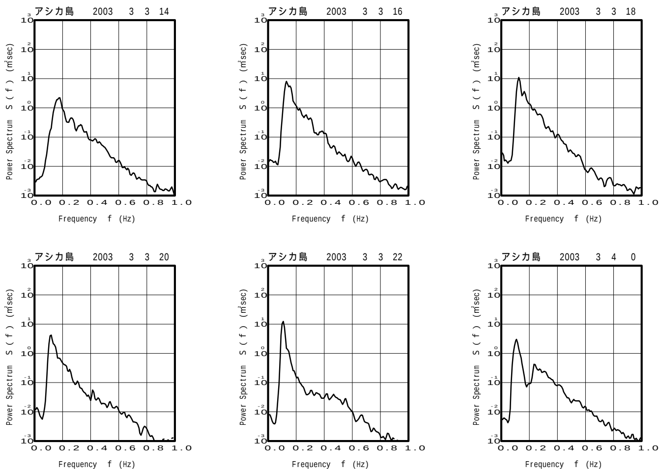
図 - 13.36 アシカ島 代表的な高波期間中のスペクトル
