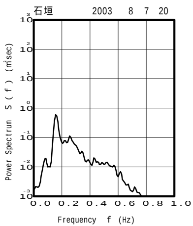
図 - 13.55 石垣 代表的な高波期間中のスペクトル
