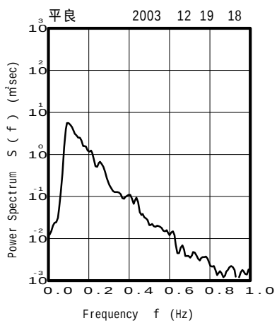
図 - 13.54 平良 代表的な高波期間中のスペクトル
