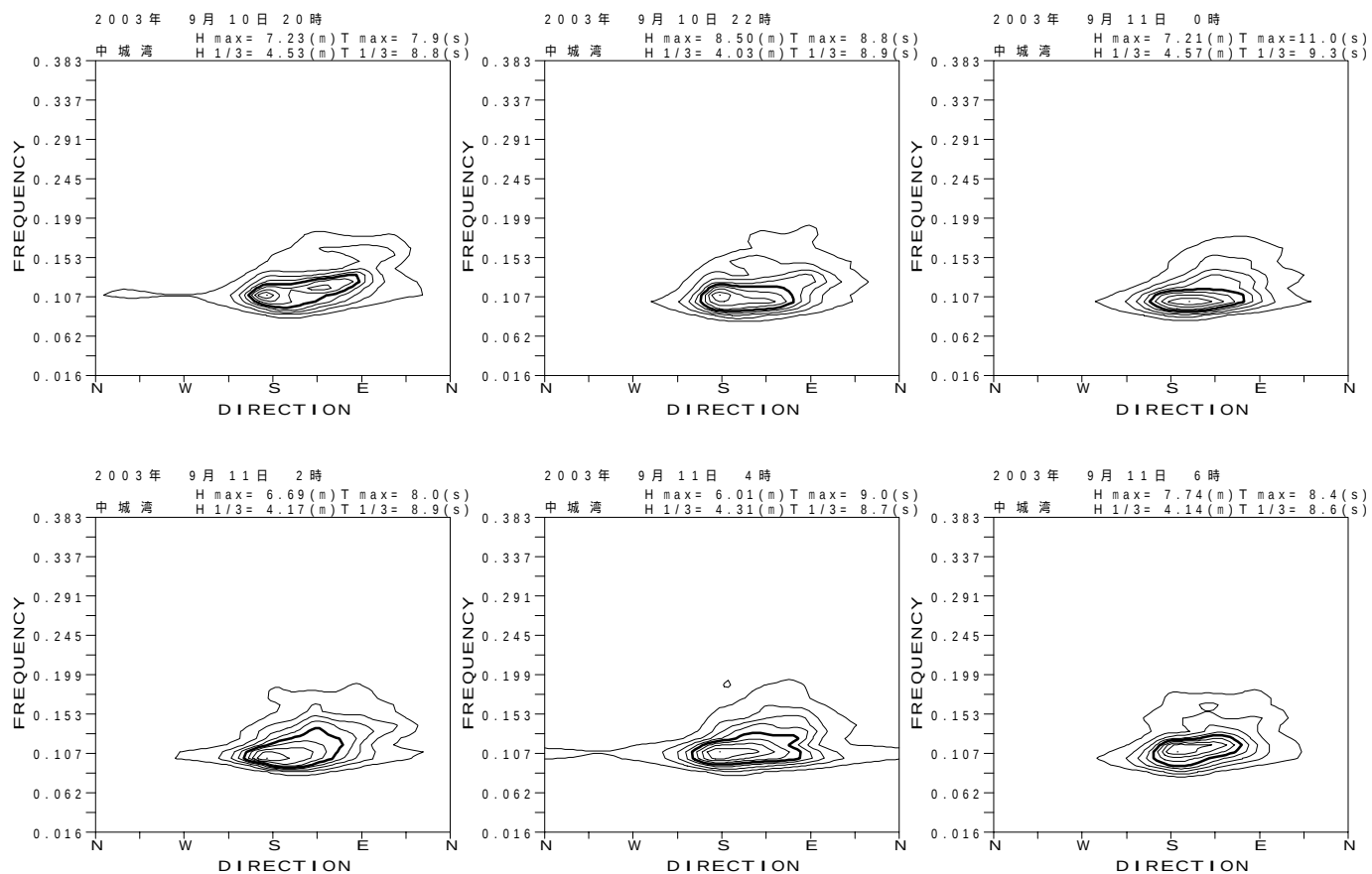
図 - 13.53 中城湾 代表的な高波期間中の方向スペクトル
