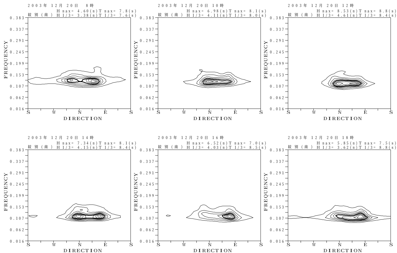
図-13.22 紋別(南) 代表的な高波期間中の方向スペクトル
