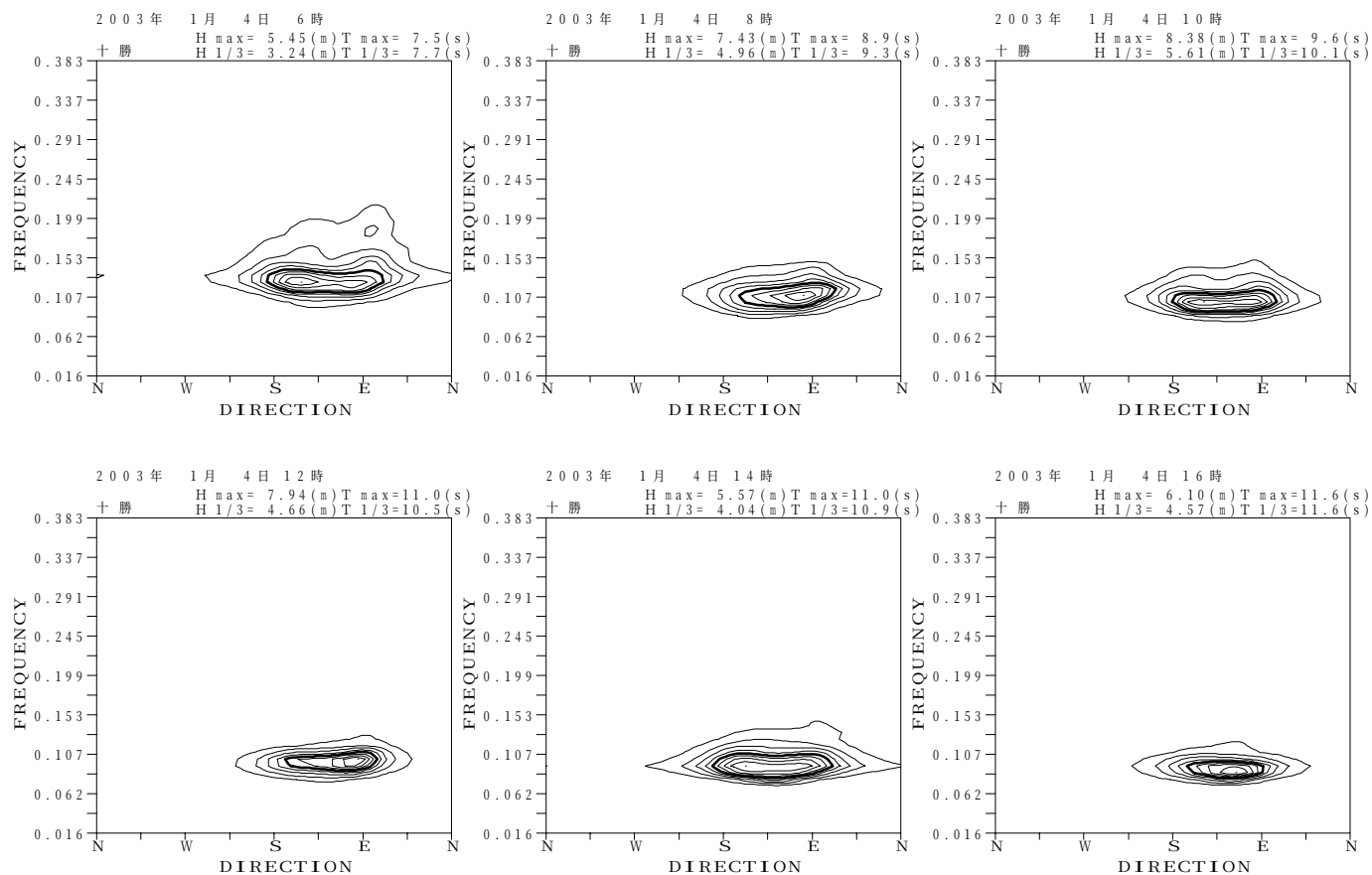
図-13.23 十勝 代表的な高波期間中の方向スペクトル
