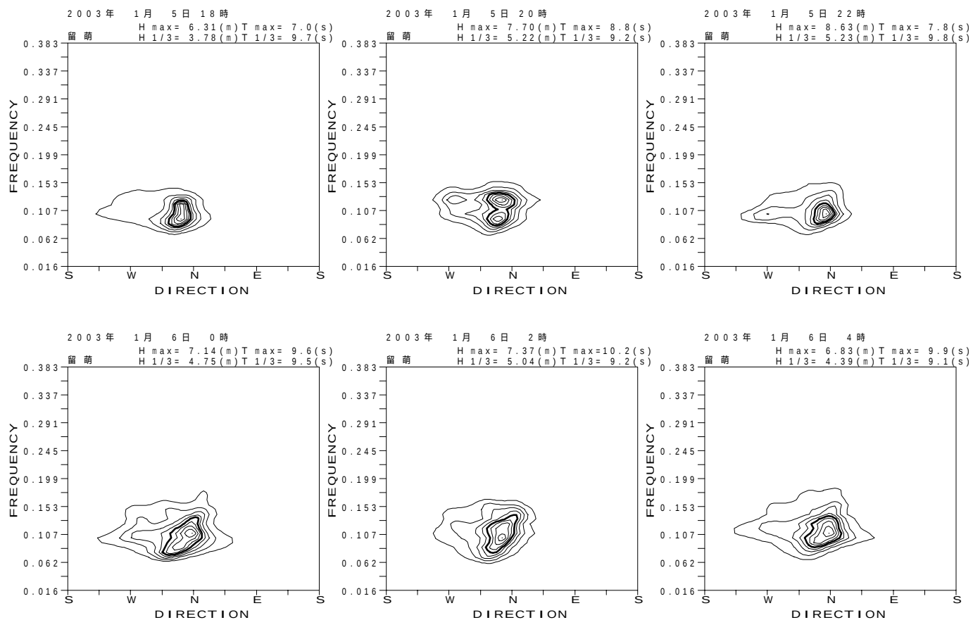
図 - 13.1 留萌 代表的な高波期間中の方向スペクトル
