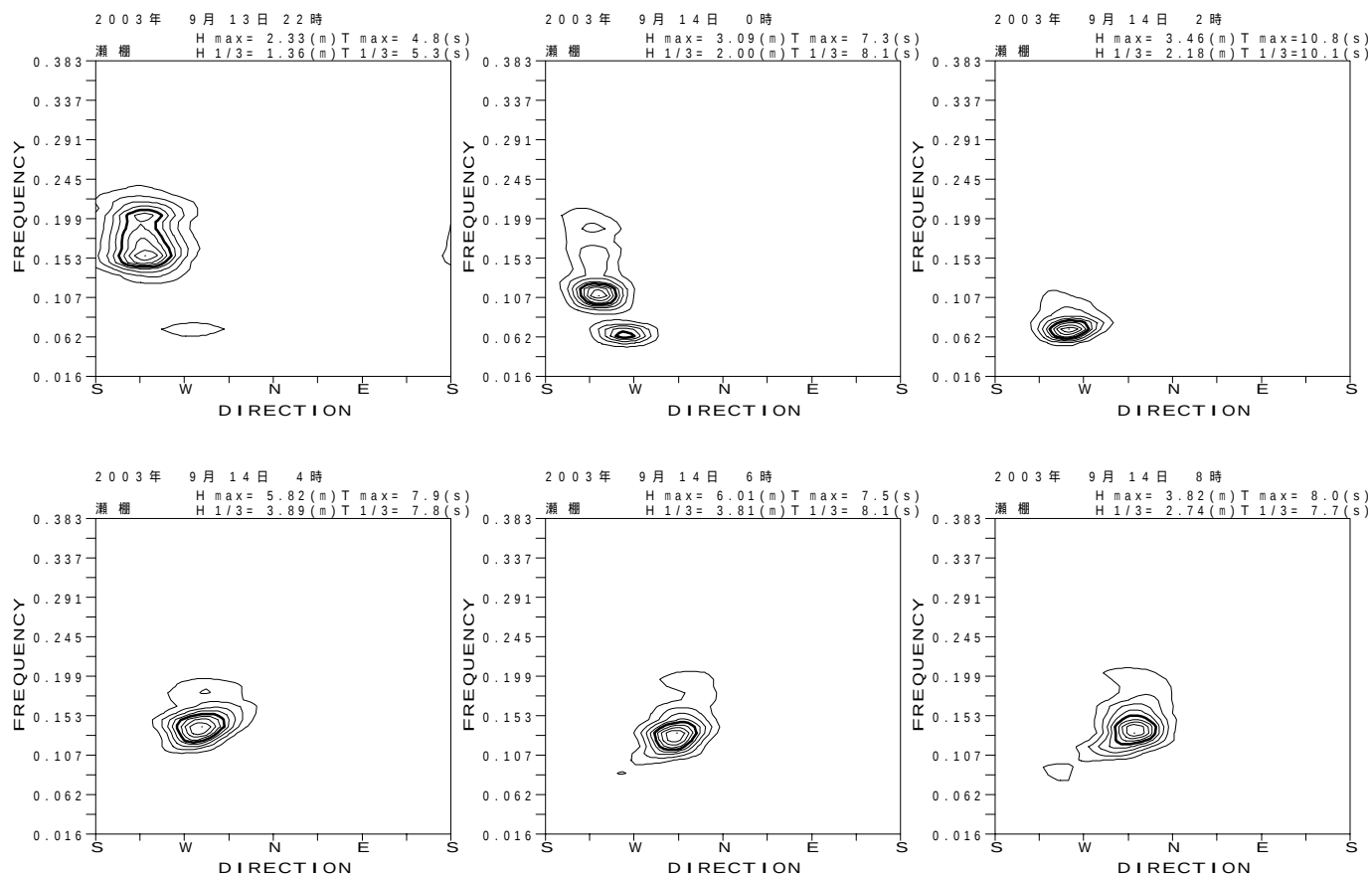
図 - 13.2 瀬棚 代表的な高波期間中の方向スペクトル
