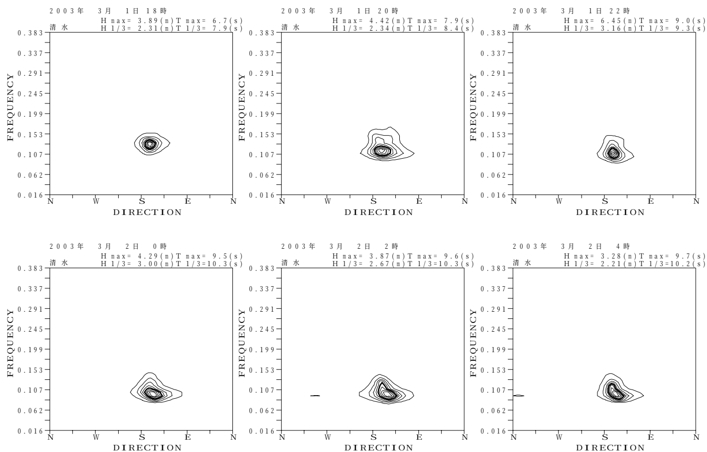
図-13.39 清水 代表的な高波期間中の方向スペクトル
