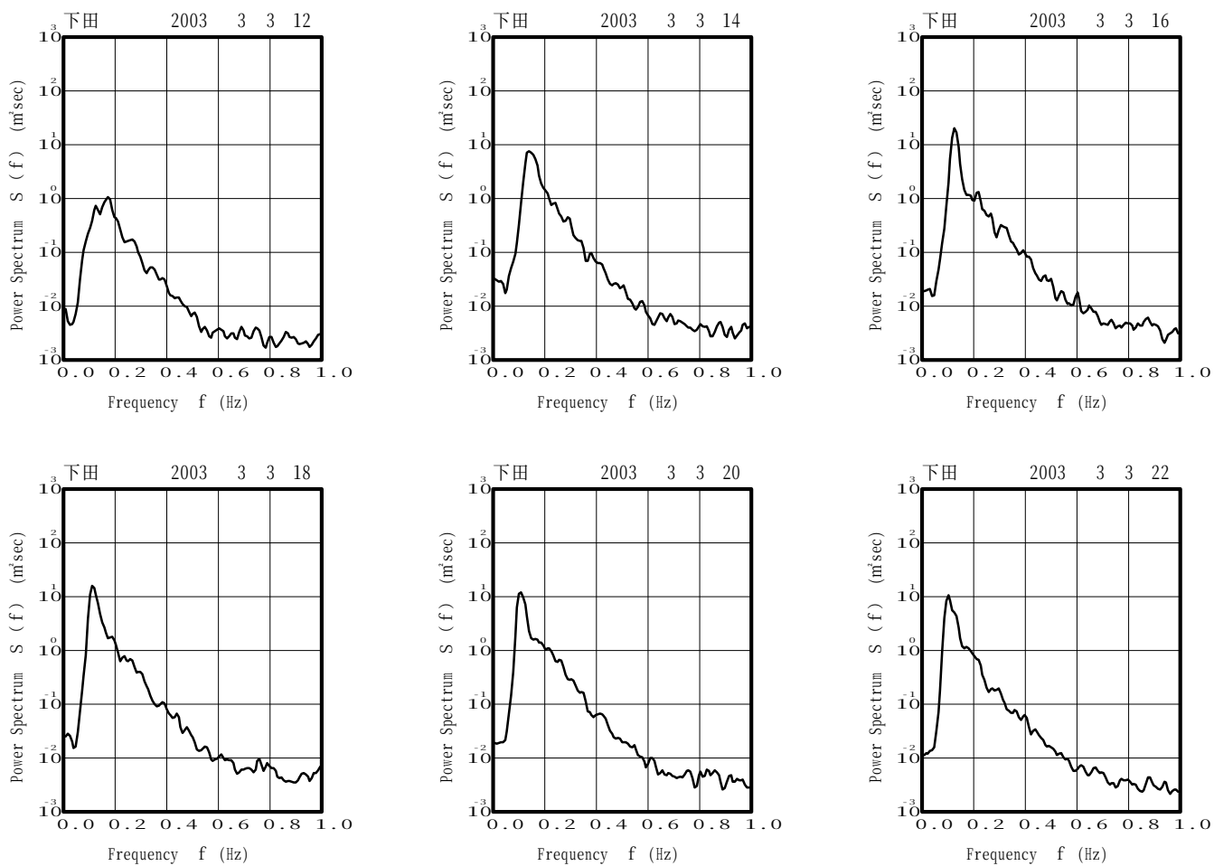
図-13.38 下田 代表的な高波期間中のスペクトル
