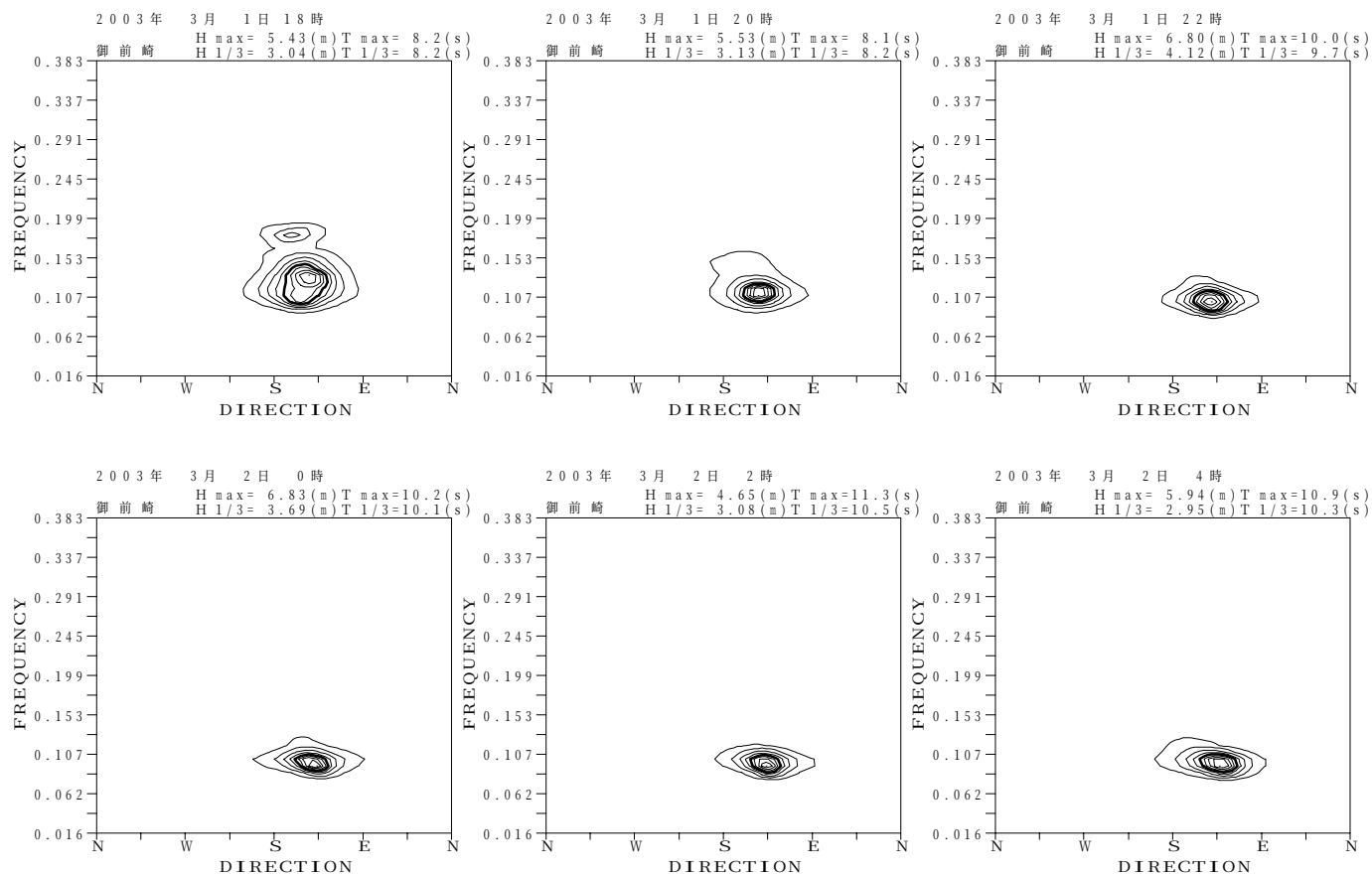
図-13.40 御前崎 代表的な高波期間中の方向スペクトル
