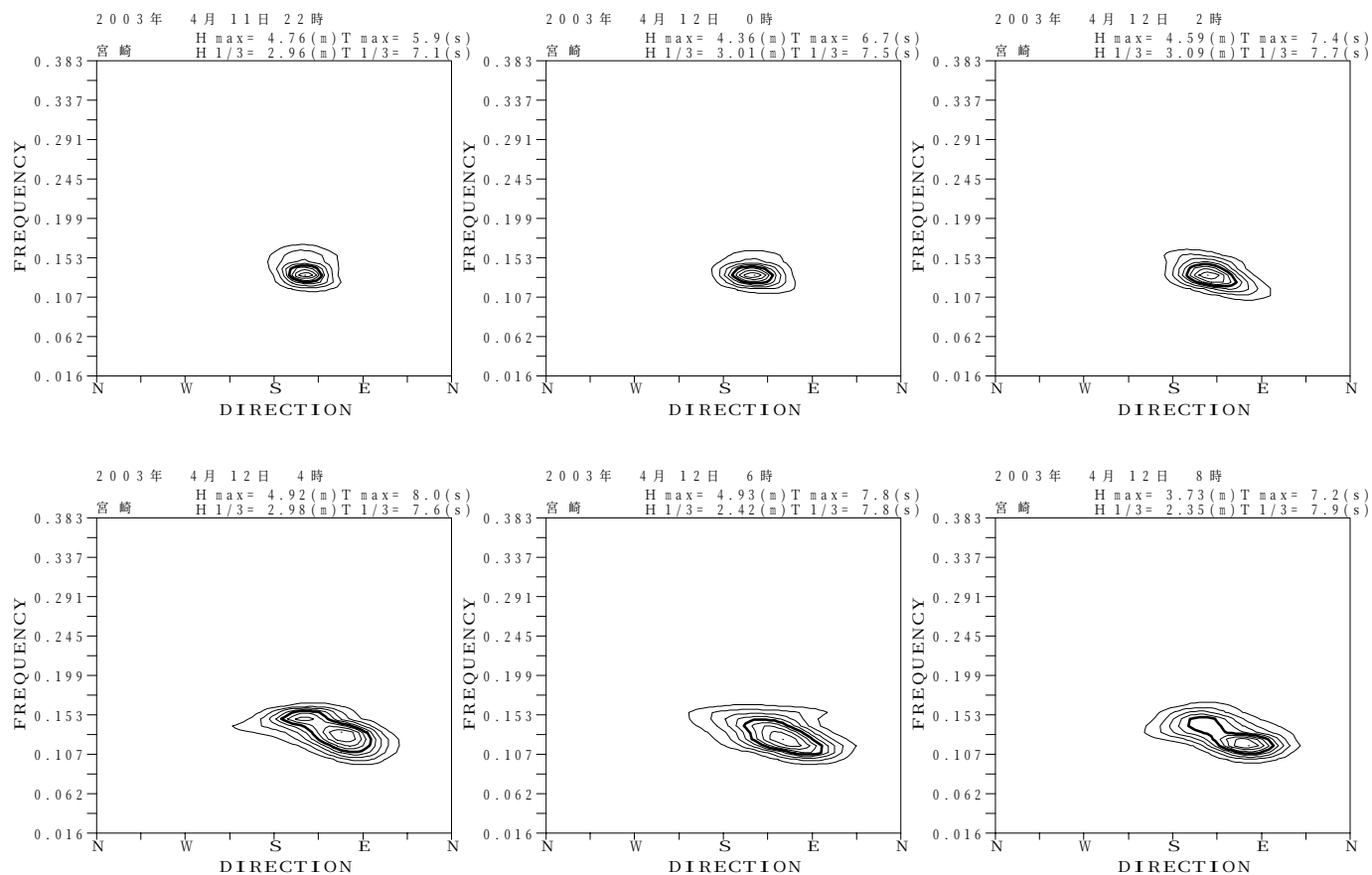
図-13.50 宮崎 代表的な高波期間中の方向スペクトル
