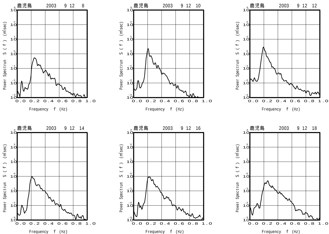
図 - 13.52 鹿児島 代表的な高波期間中のスペクトル
