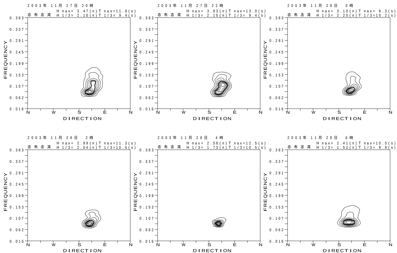
図 - 13.51 志布志湾 代表的な高波期間中の方向スペクトル
