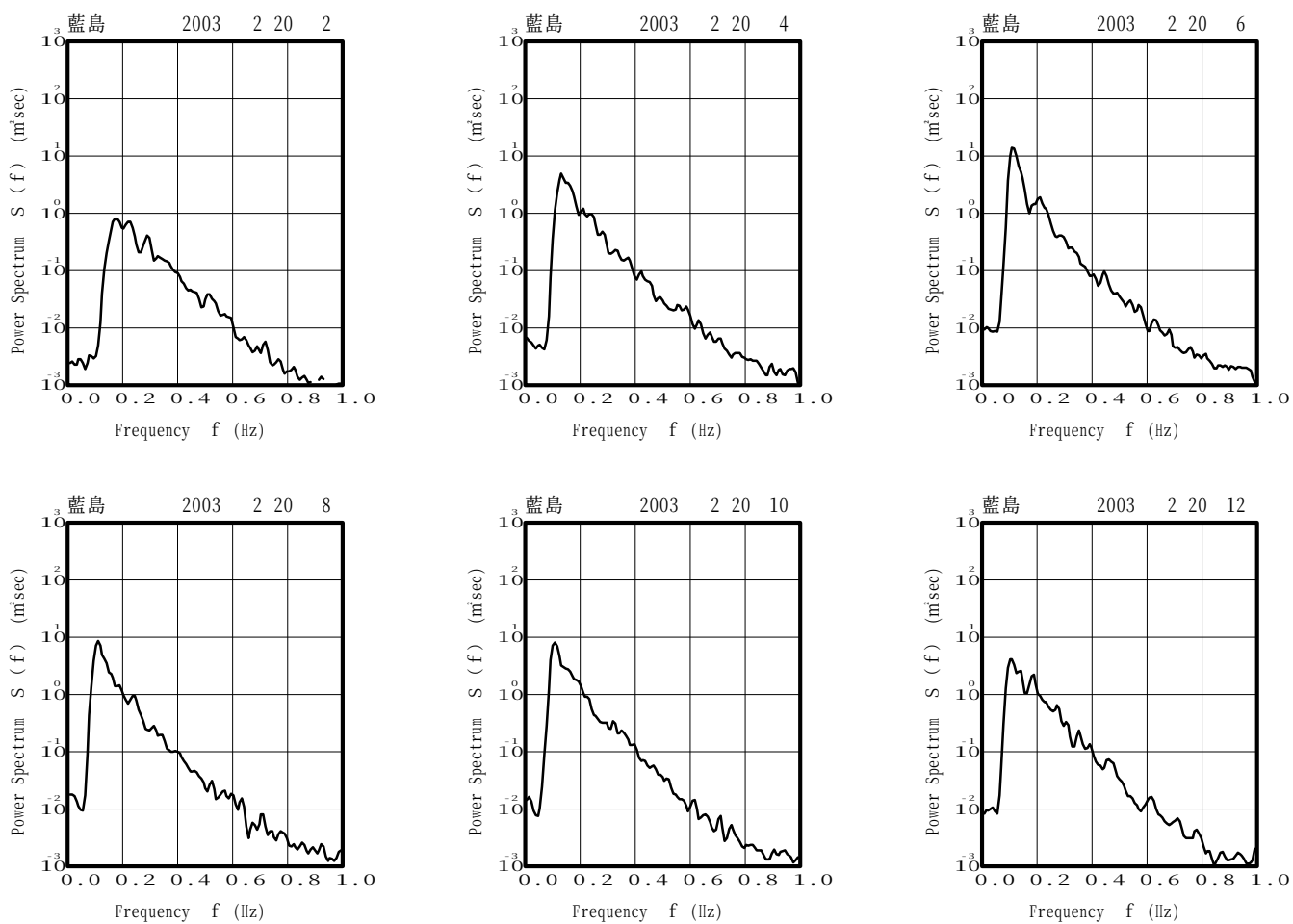
図-13.17 藍島 代表的な高波期間中のスペクトル
