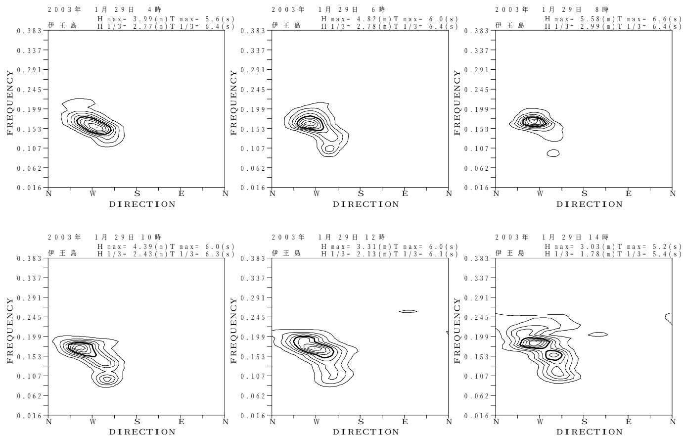
図-13.19 伊王島 代表的な高波期間中の方向スペクトル
