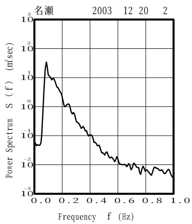
図-13.20 名瀬 代表的な高波期間中のスペクトル
