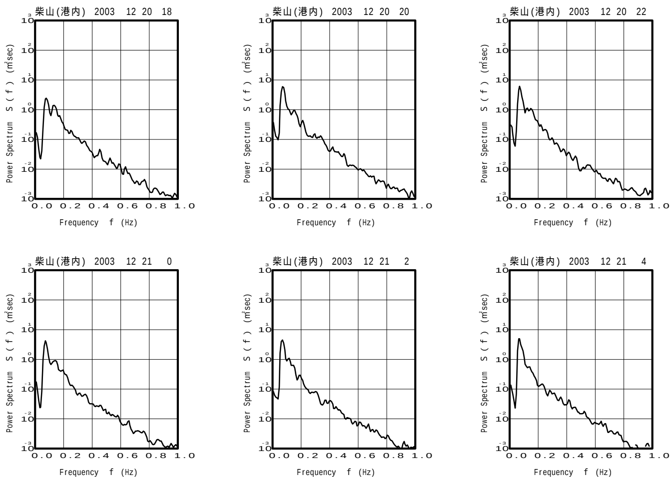
図 - 13.13 柴山(港内) 代表的な高波期間中のスペクトル
